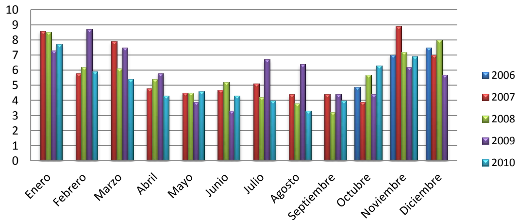
Gráfica No. 1 Velocidades de viento promedio mensual en m/s, a 30 m Durazno, Jutiapa, Jutiapa
