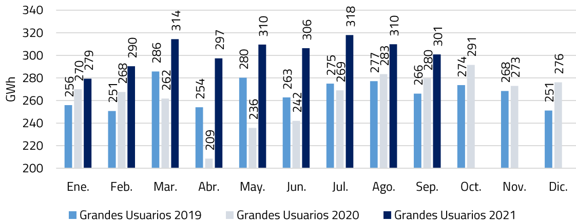
Demanda de energía mensual de G.U.
