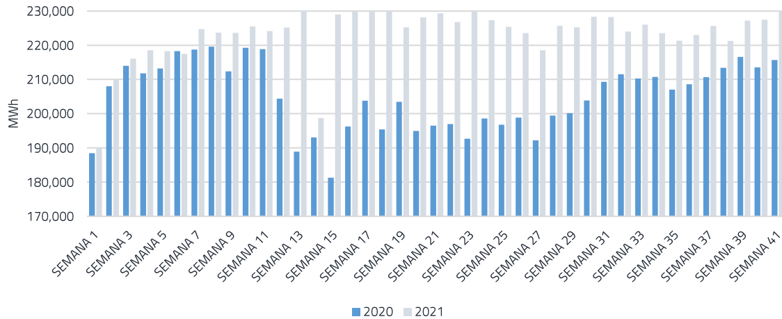
Demanda de energía semanal del SNI 2020 y 2021
