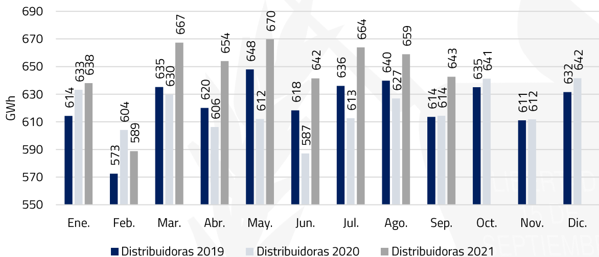
Demanda de energía mensual de A.D.
