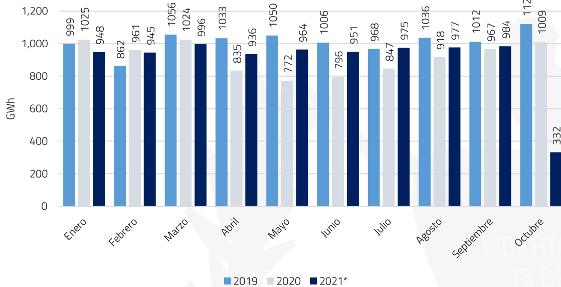
Generación mensual SNI
