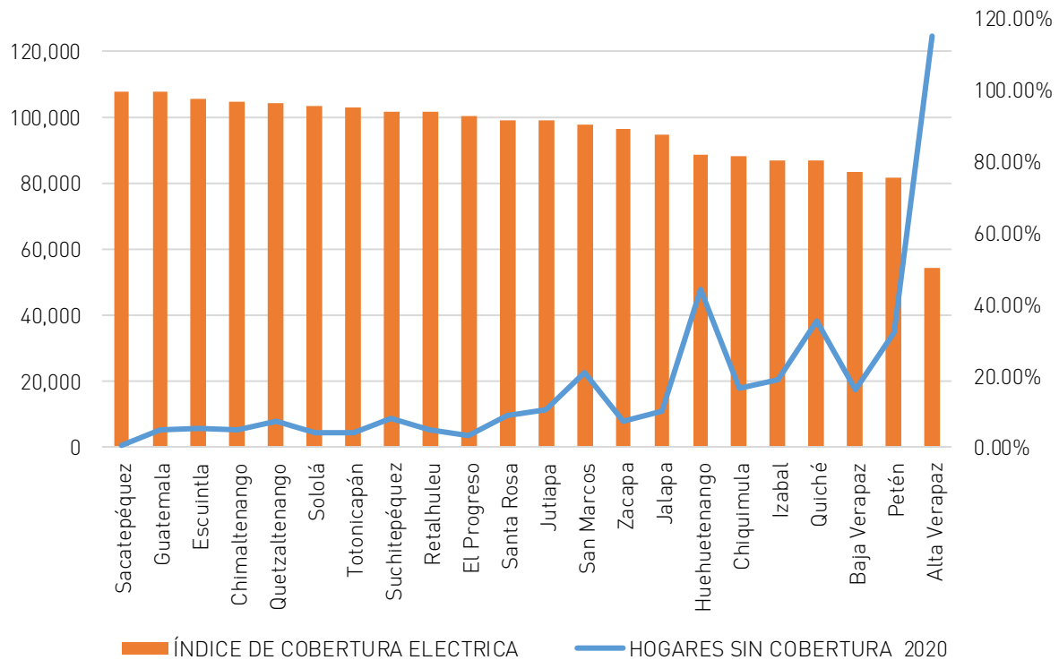
Gráfica 2: Índice de Cobertura Eléctrica y cantidad de hogares sin cobertura eléctrica.
