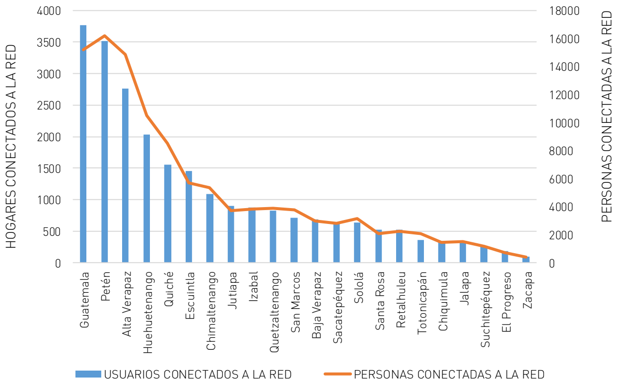
Gráfica 3: Hogares Electrificados.
