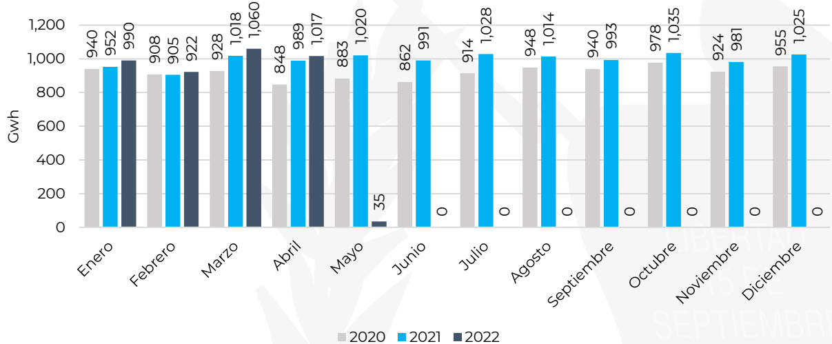
Demanda de energía mensual del SNI
