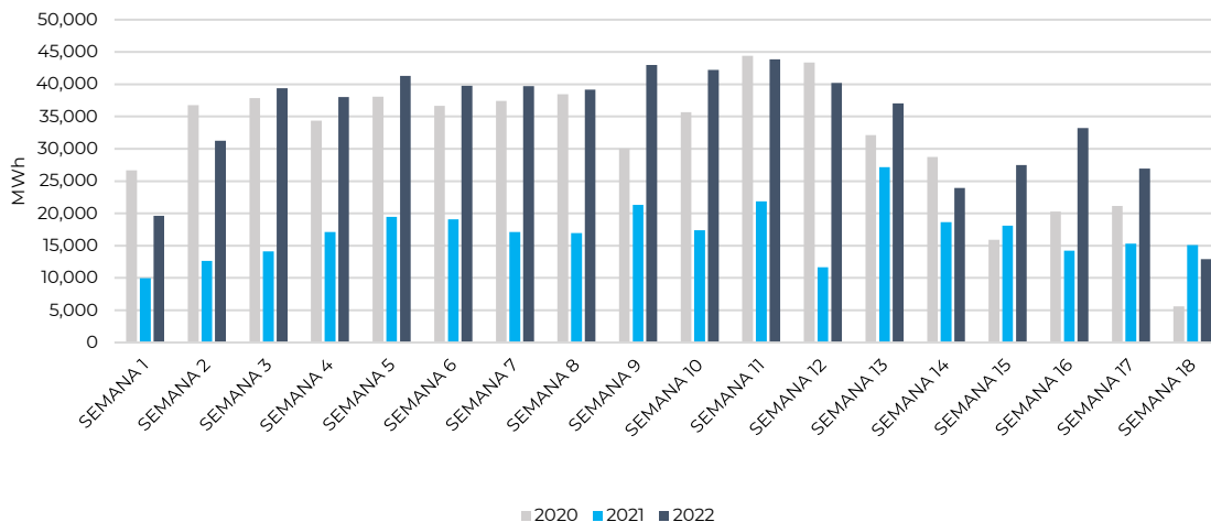
Intercambios de energía netos por semana con el Mercado Eléctrico Regional
