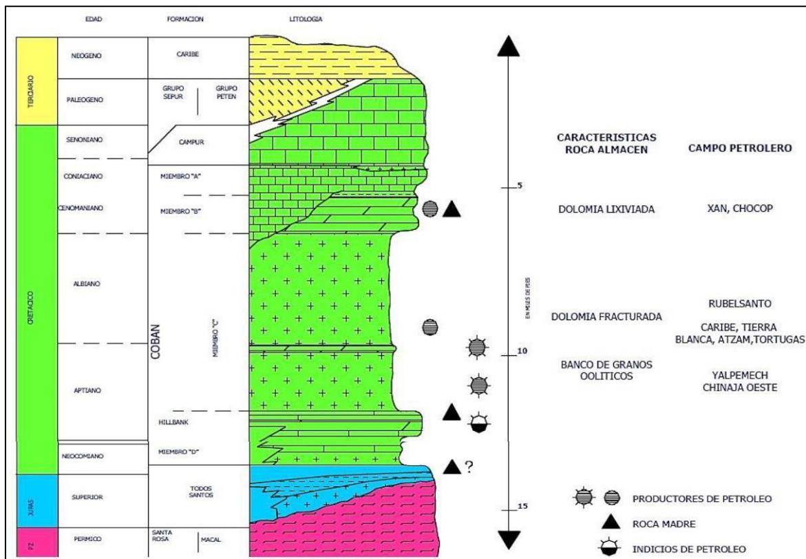
Figura 2. Estratigrafía Generalizada de la Cuenca Petén. Departamento de Exploración.
