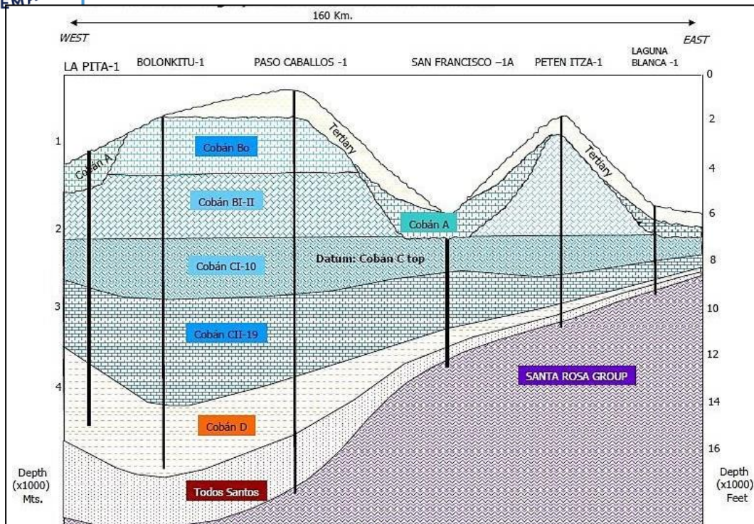
Figura 5. Sección Estratigráfica transversal de la subcuenca Petén Norte. Departamento de Exploración.
