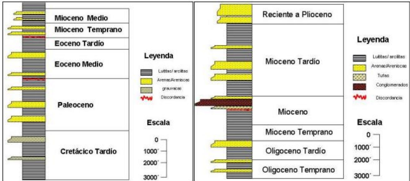
Figura 13. Columna estratigráfica de pozos Petrel-1 y Madre Vieja-1 ubicados en la Cuenca Pacífico. Departamento de Exploración
