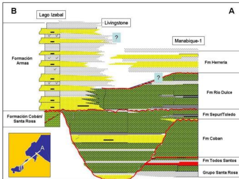
Figura 10. Esquema de variabilidad estratigráfica de la cuenca de Izabal. Departamento de Exploración
