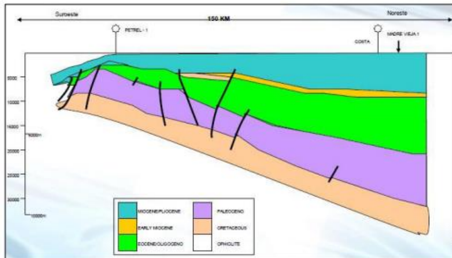
Figura 12. Perfil de la cuenca Pacifico. Departamento de Exploración.
