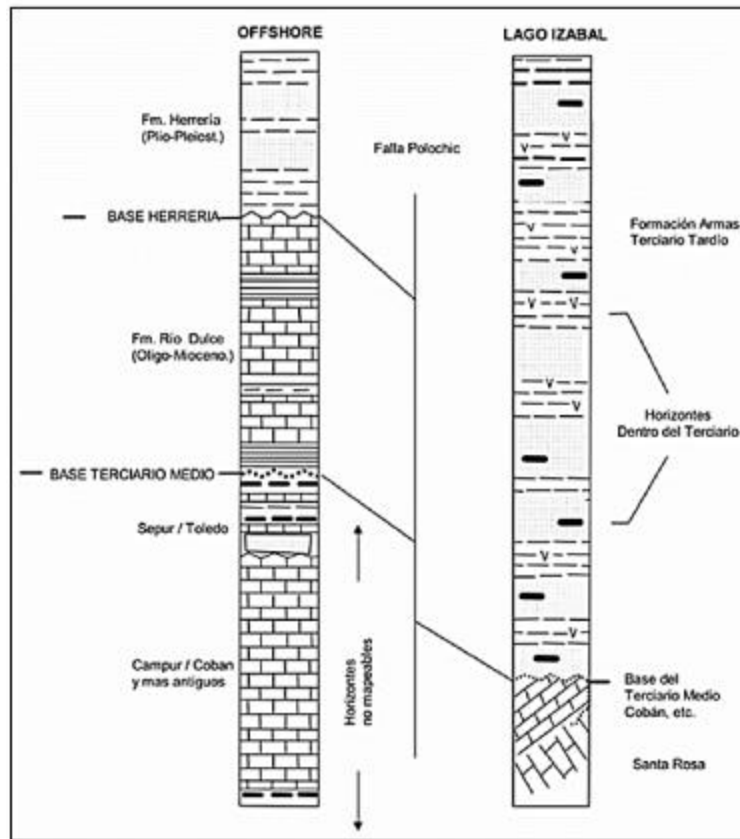
Figura 9. Columna Litoestratigráfica Cuenca de Amatique. Departamento de Exploración
