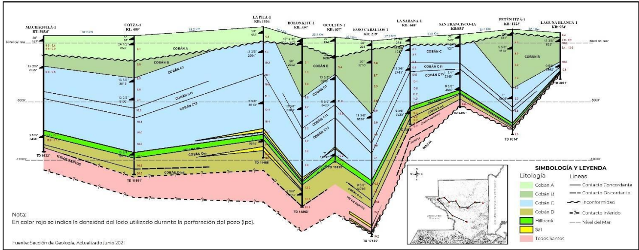
Figura 7. Correlación Estratigráfica de la Cuenca Petén. Departamento de Exploración.
