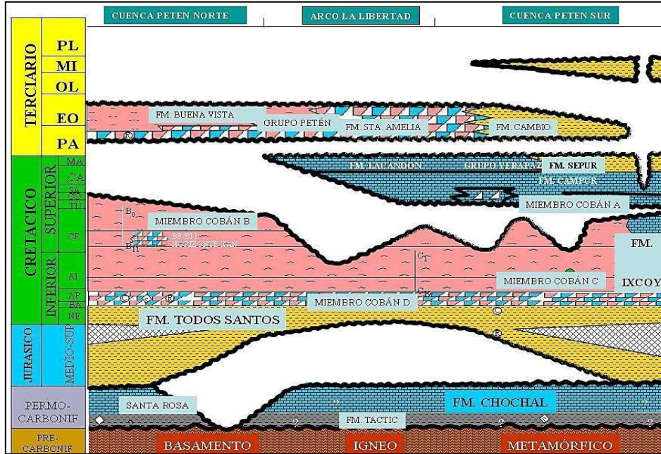
Figura 3. Correlación Estratigráfica entre las subcuencas Petén Norte y Sur. Departamento de Exploración.
