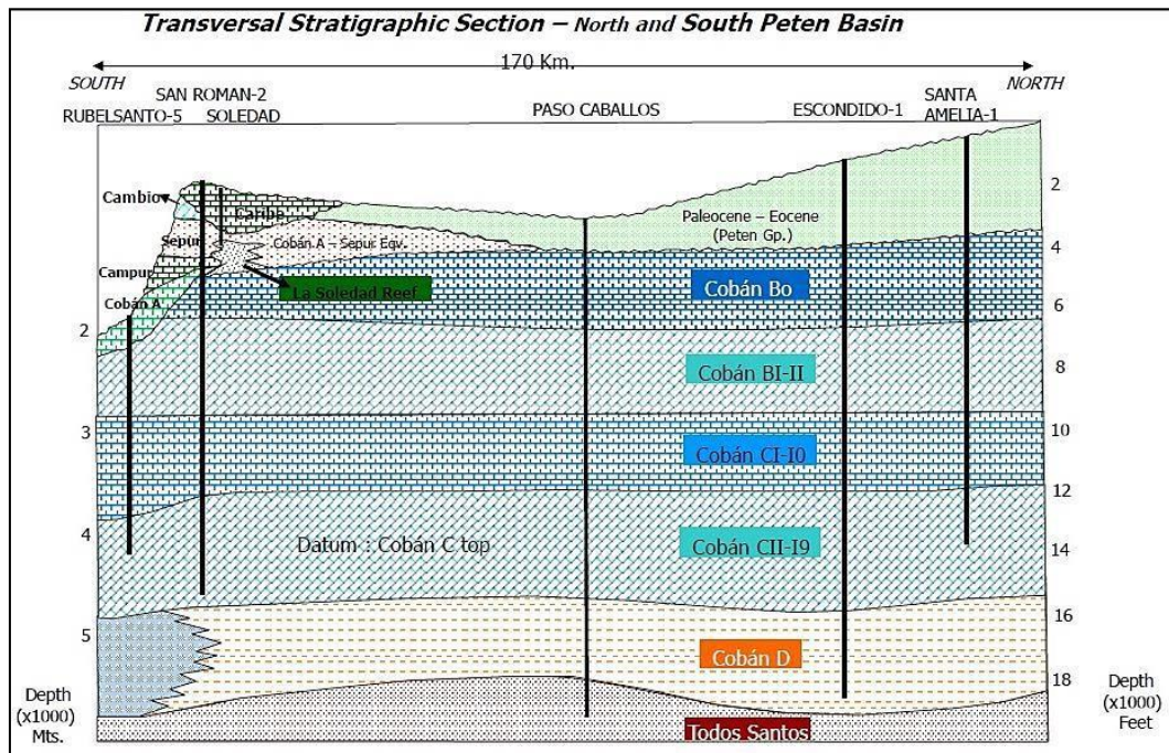
Figura 4. Sección Estratigráfica de las subcuencas Petén Norte y Petén Sur. Departamento de Exploración.
