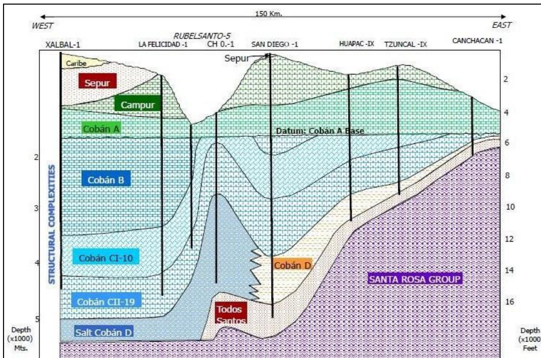
Figura 6. Sección Estratigráfica Transversal de la subcuenca Petén Sur. Departamento de Exploración.
